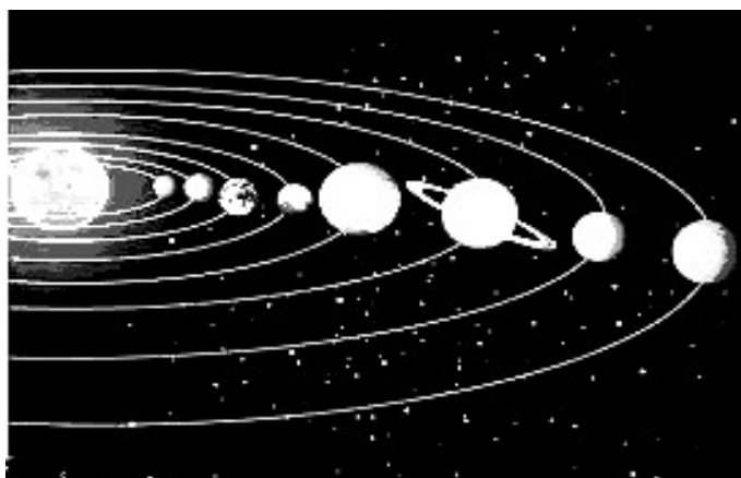
图 1 太阳系
